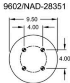
PISTON BOTTOM
